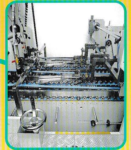
ロックボトムセクション (ワンタッチ昇降式)
