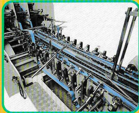
メインフォルディングセクション (脱着式中レール付)
